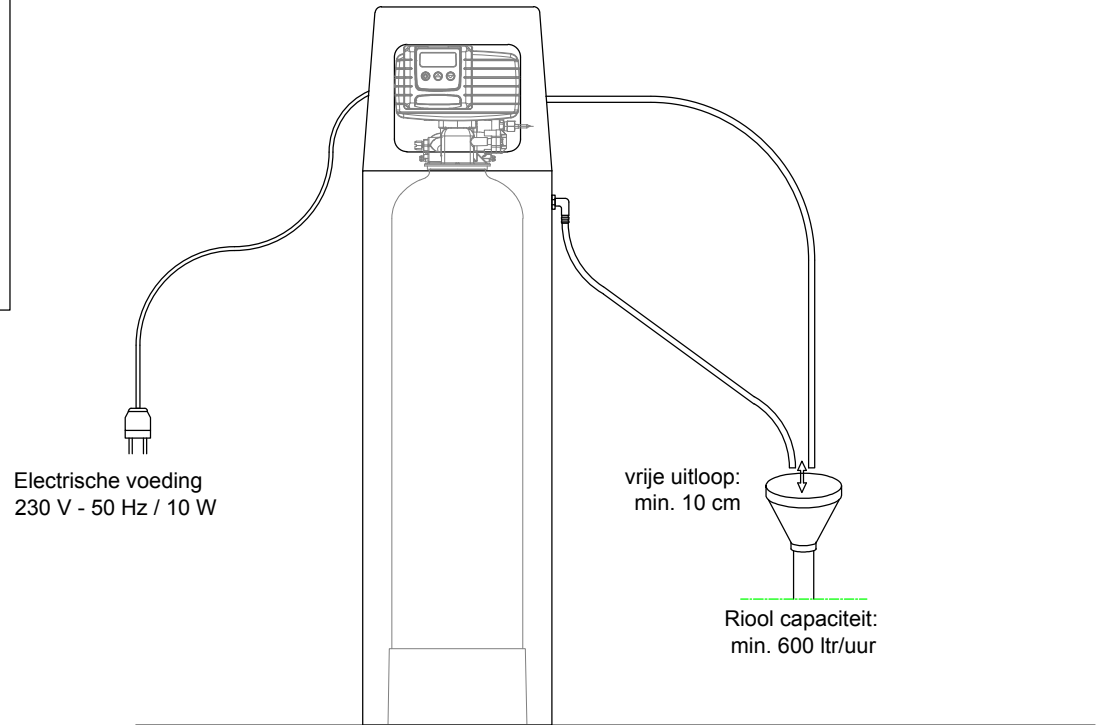
Vooraanzicht
