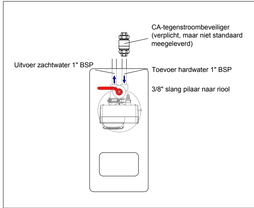
Bovenaanzicht
