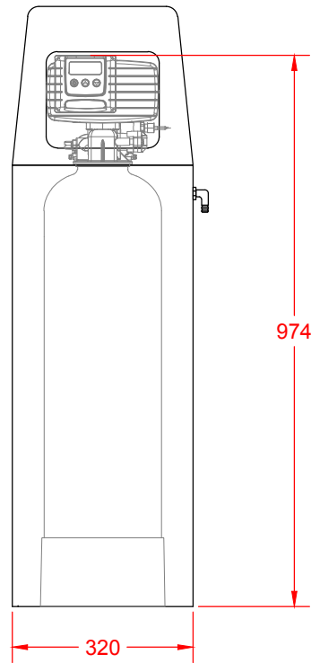
vooraanzicht
