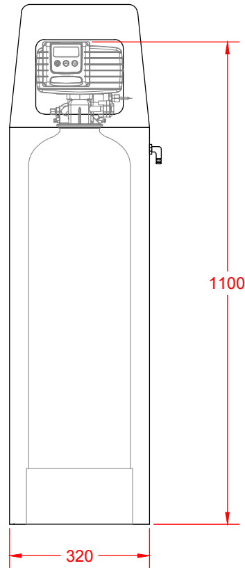
vooraanzicht
