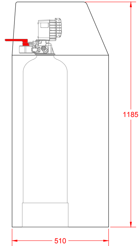
zijaanzicht
