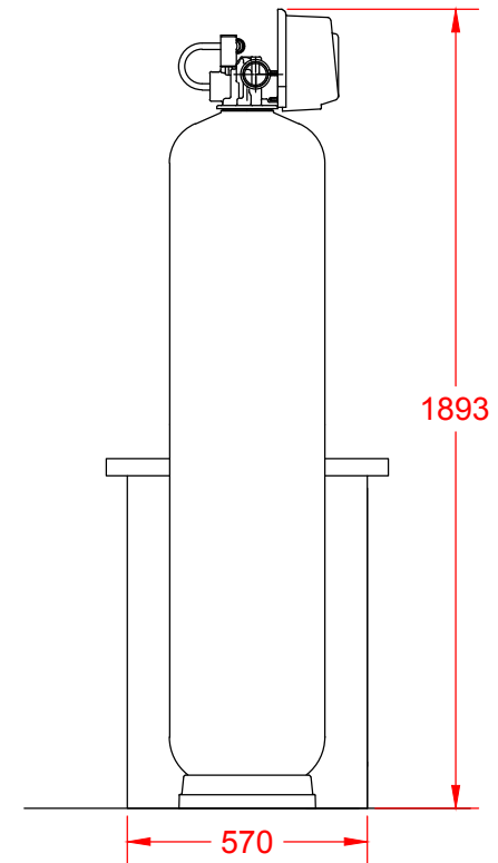
Zijaanzicht
