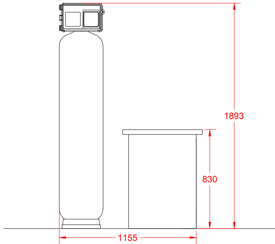
Vooraanzicht
