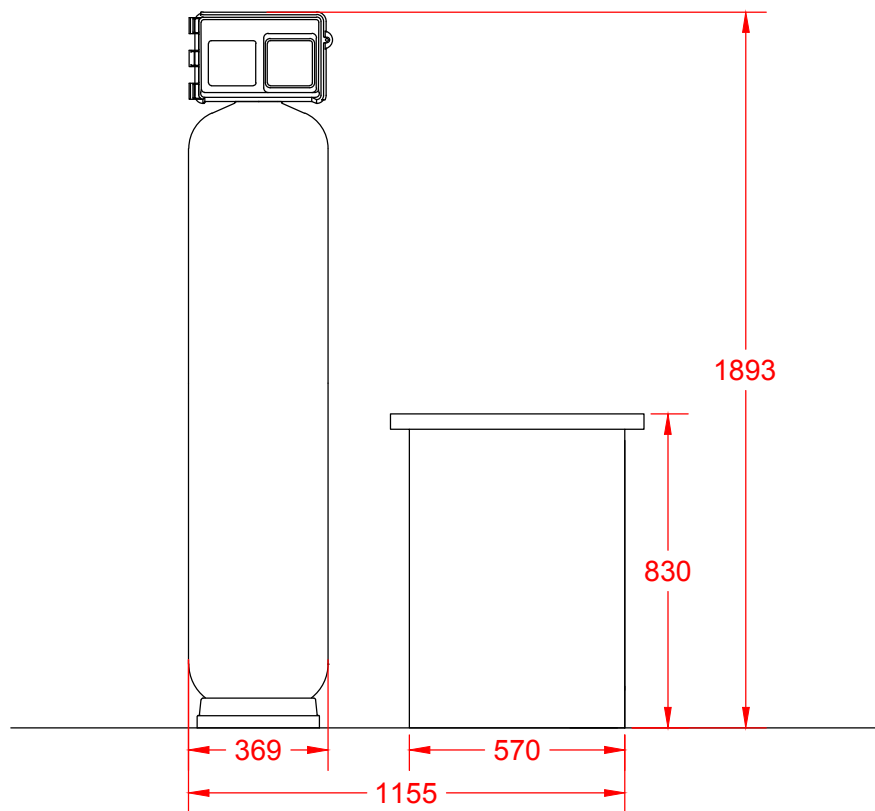
Vooraanzicht
