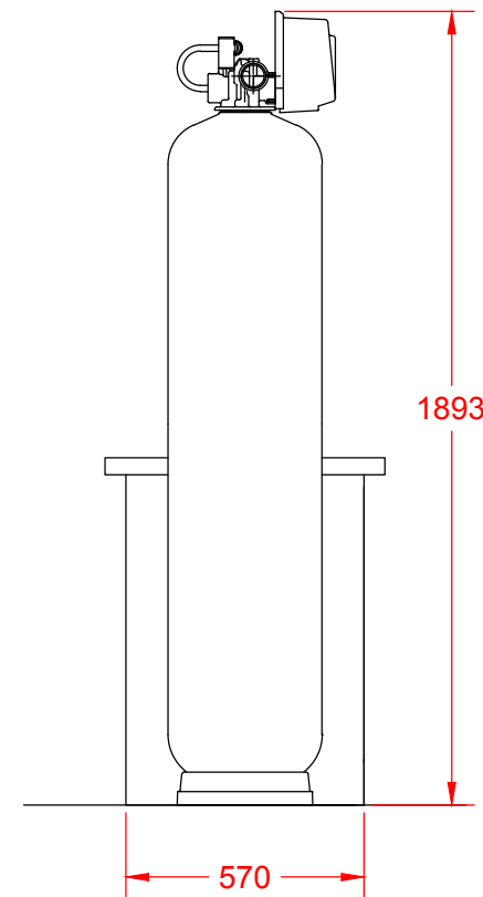
Zijaanzicht
