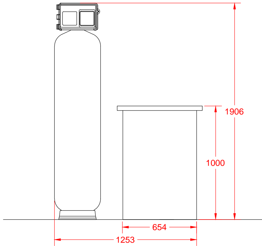
Vooraanzicht
