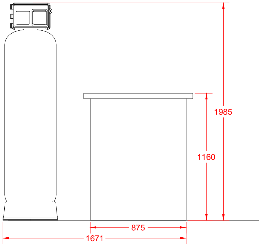
Vooraanzicht
