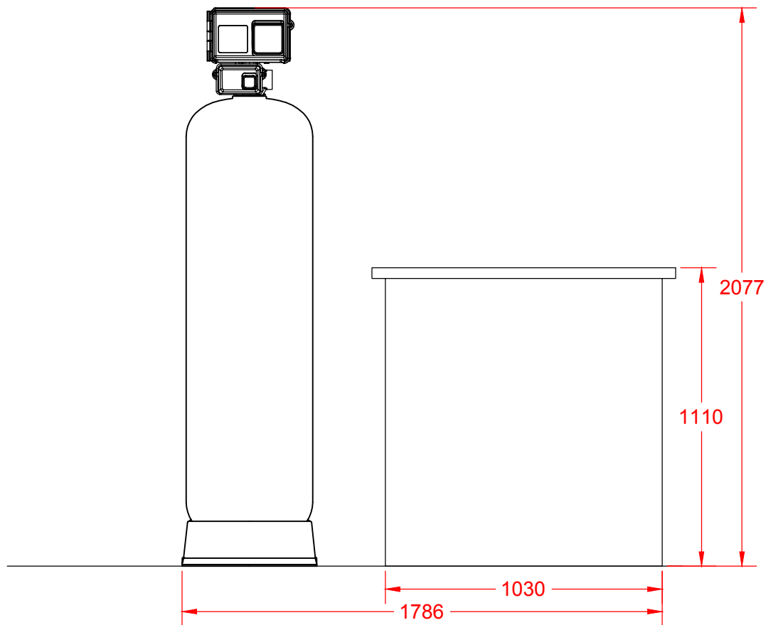
Vooraanzicht
