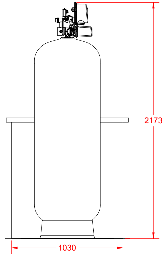
Zijaanzicht
