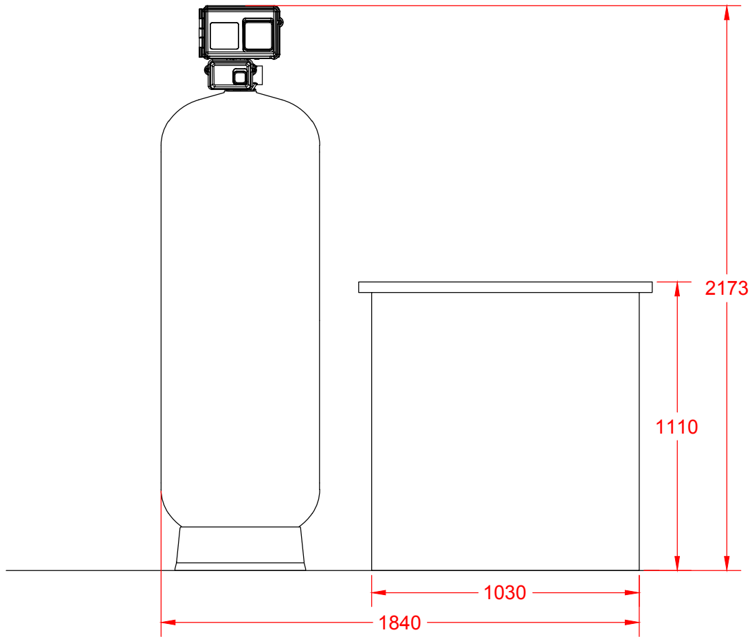
Vooraanzicht
