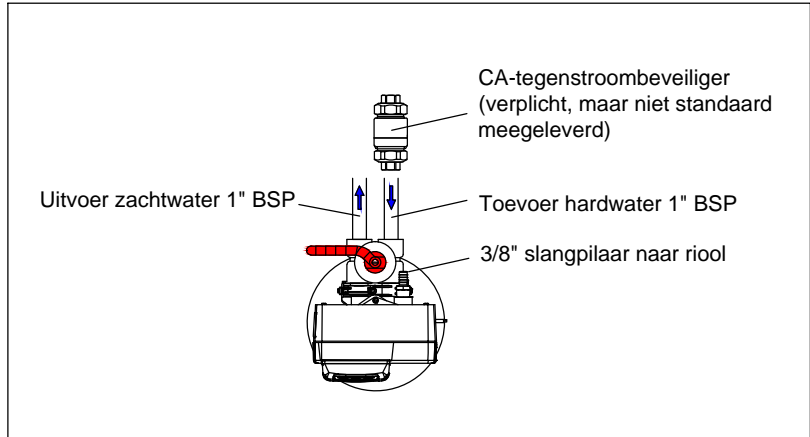
Bovenaanzicht
