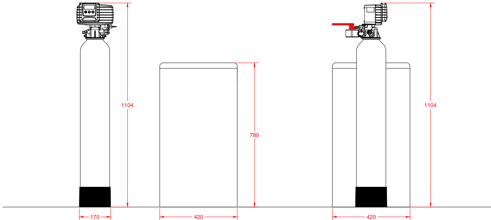
Vooraanzicht
