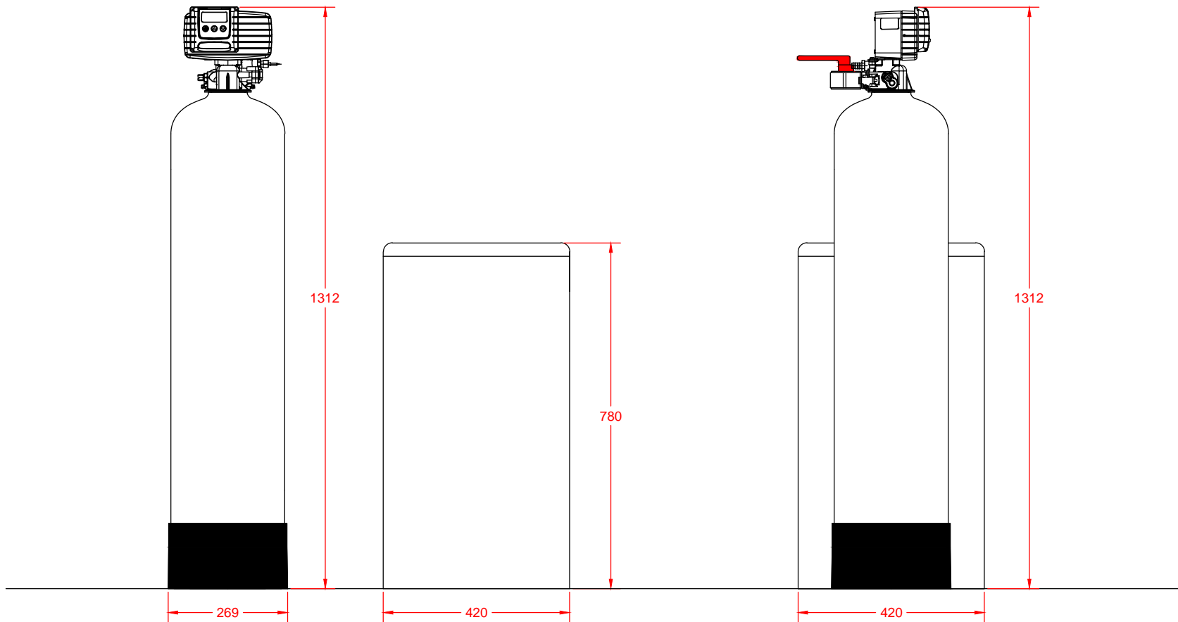
Zijaanzicht
