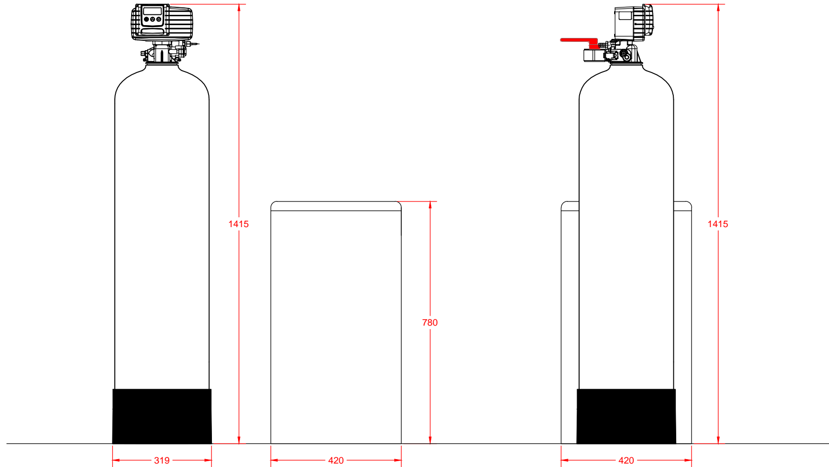
Vooraanzicht
