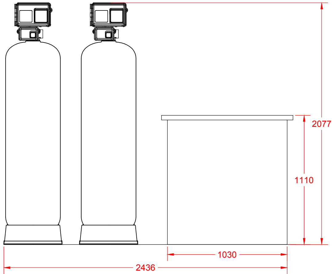
Vooraanzicht
