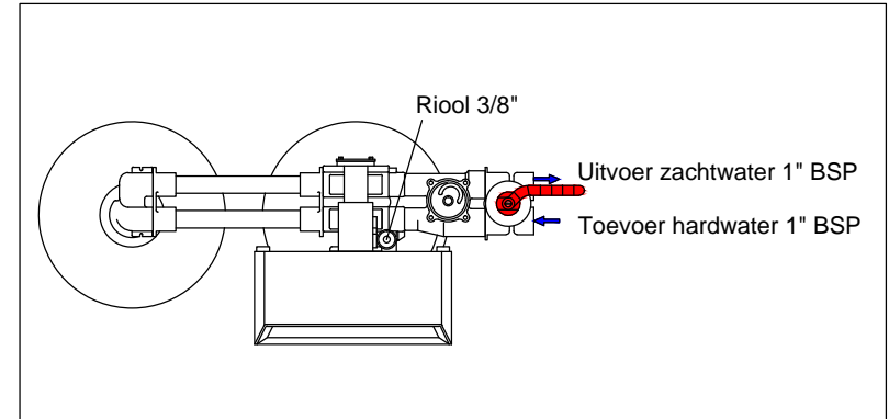
Bovenaanzicht
