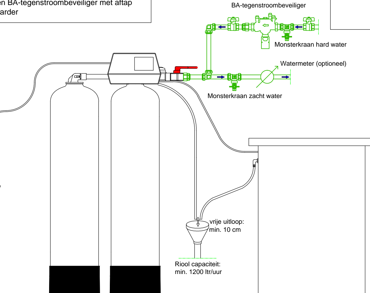
Vooraanzicht
