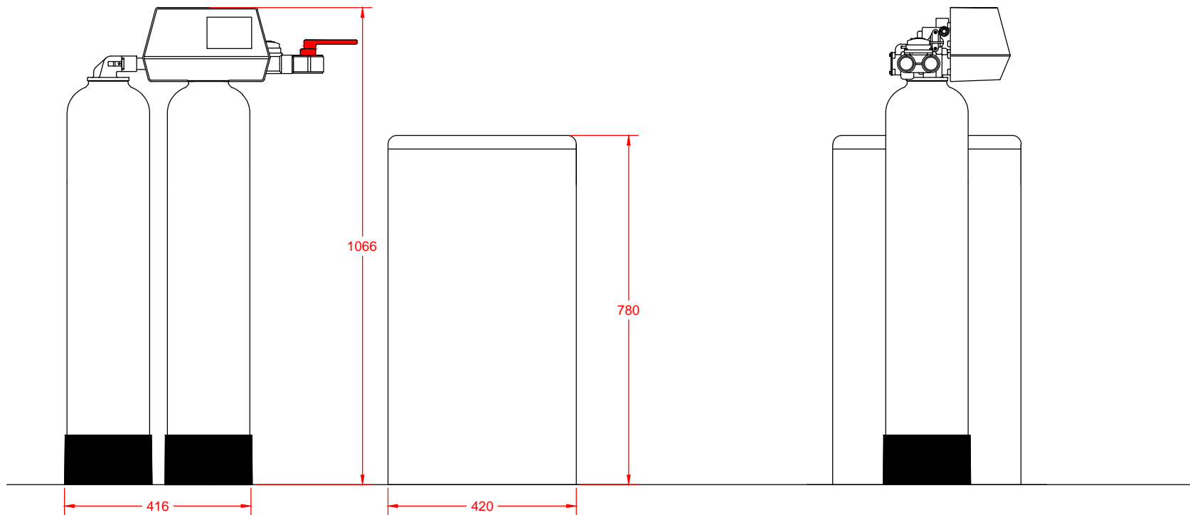
Vooraanzicht
