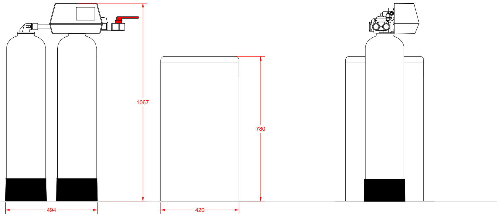
Zijaanzicht
