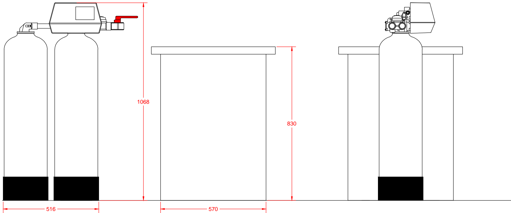
Vooraanzicht
