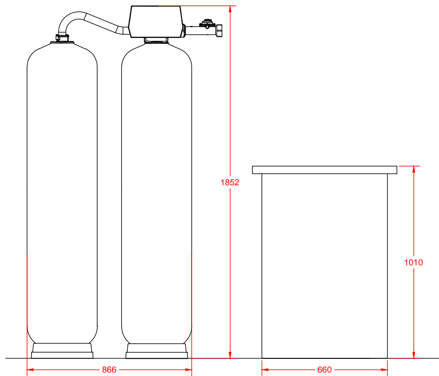
Vooraanzicht
