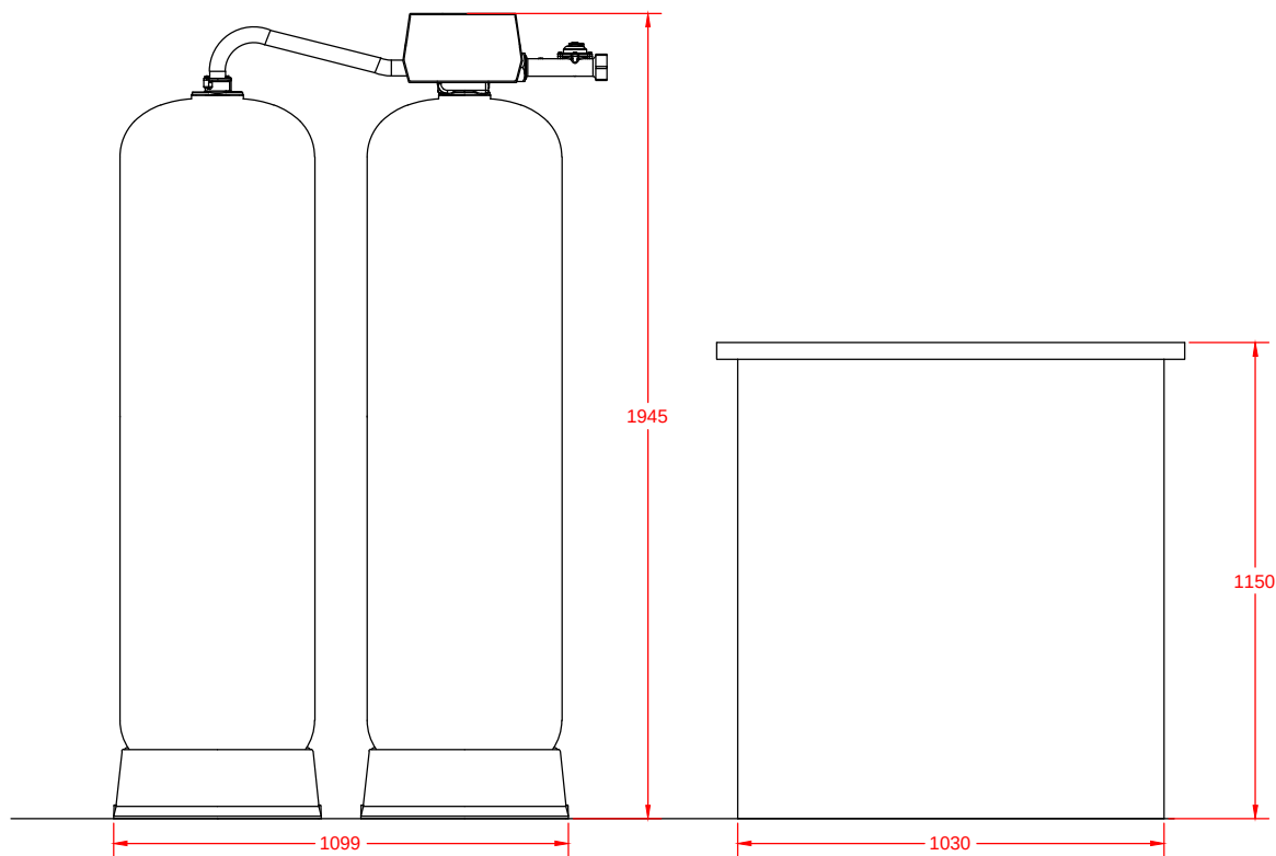
Vooraanzicht
