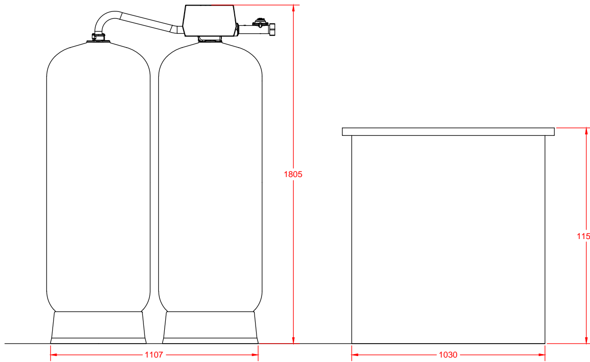
Vooraanzicht
